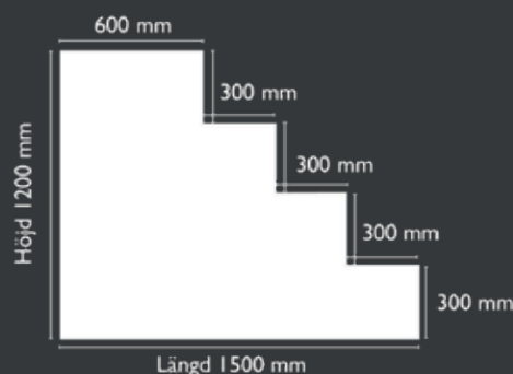
Ritningen visar gavel- och helgaveltrappa med fyra trappsteg, sett rakt från sidan
