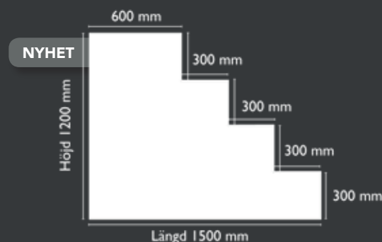
Ritningen visar gavel- och helgaveltrappa med fyra trappsteg, sett rakt från sidan
