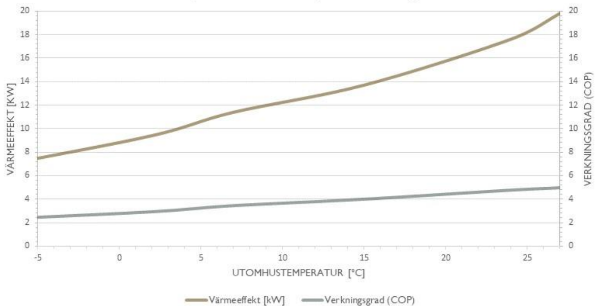
Värmeeffekt [kW] och verkningsgrad (COP) för S40-3P beroende på utomhustemperatur enligt NF 414
