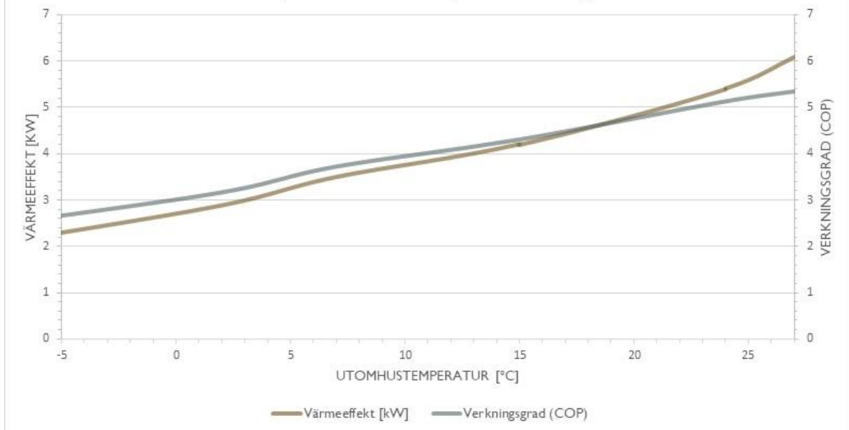
Värmeeffekt [kW] och verkningsgrad (COP) för S15 beroende på utomhustemperatur enligt NF 414
