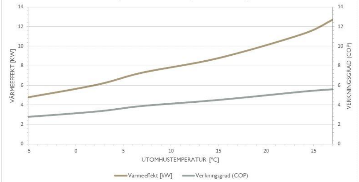
Värmeeffekt [kW] och verkningsgrad (COP) för S30-3P beroende på utomhustemperatur enligt NF 414
