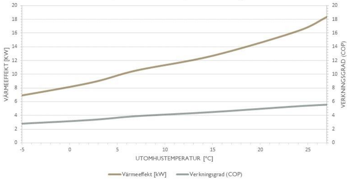
Värmeeffekt [kW] och verkningsgrad (COP) för S40 beroende på utomhustemperatur enligt NF 414
