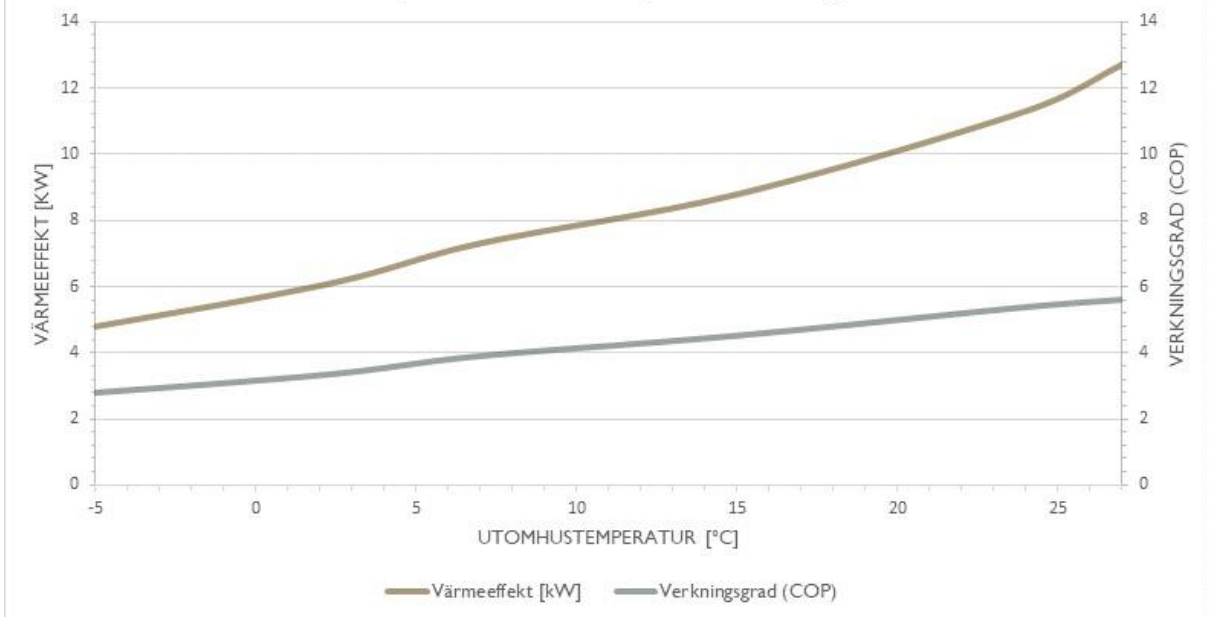
Värmeeffekt [kW] och verkningsgrad (COP) för S30 beroende på utomhustemperatur enligt NF 414
