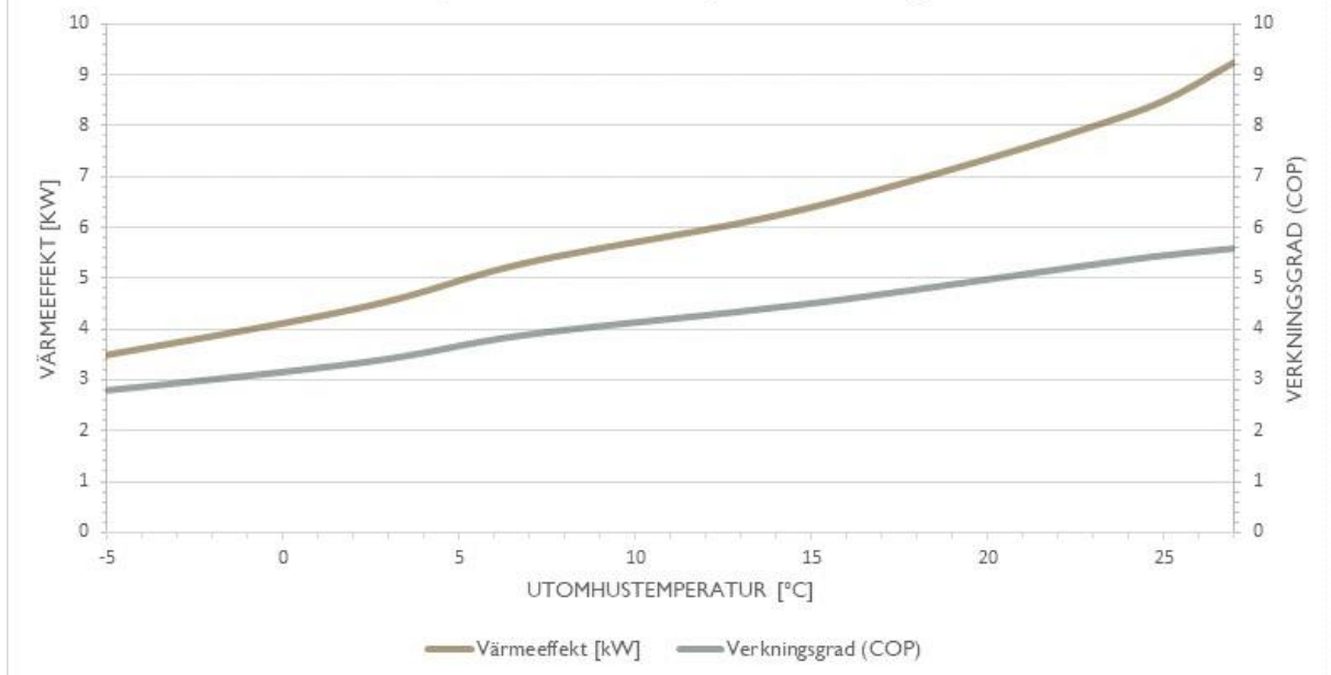
Värmeeffekt [kW] och verkningsgrad (COP) för S20 beroende på utomhustemperatur enligt NF 414
