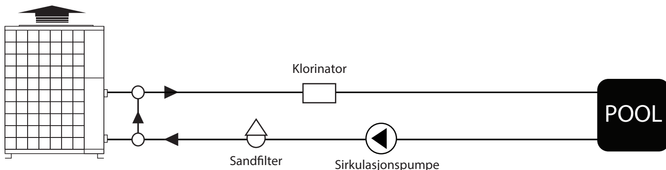
Prinsippkisse for installasjon av X-serien
